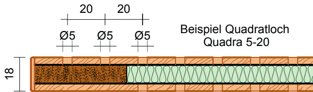
Tür-Element / Orbit oder Quadra / Standard
