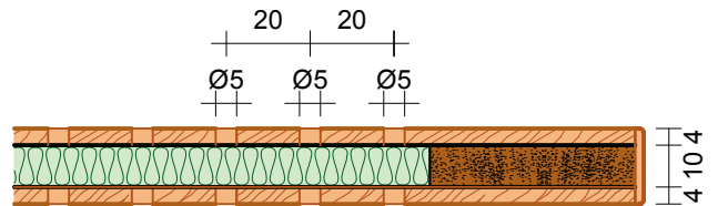
Tür-Element / Orbit oder Quadra / variabel
